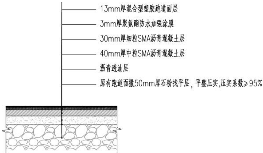
图 1—跑道及半圆区结构图
