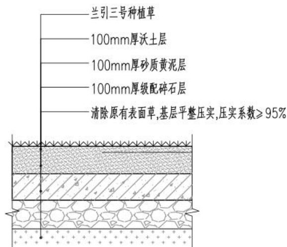
图 2—足球场草坪改造结构图
